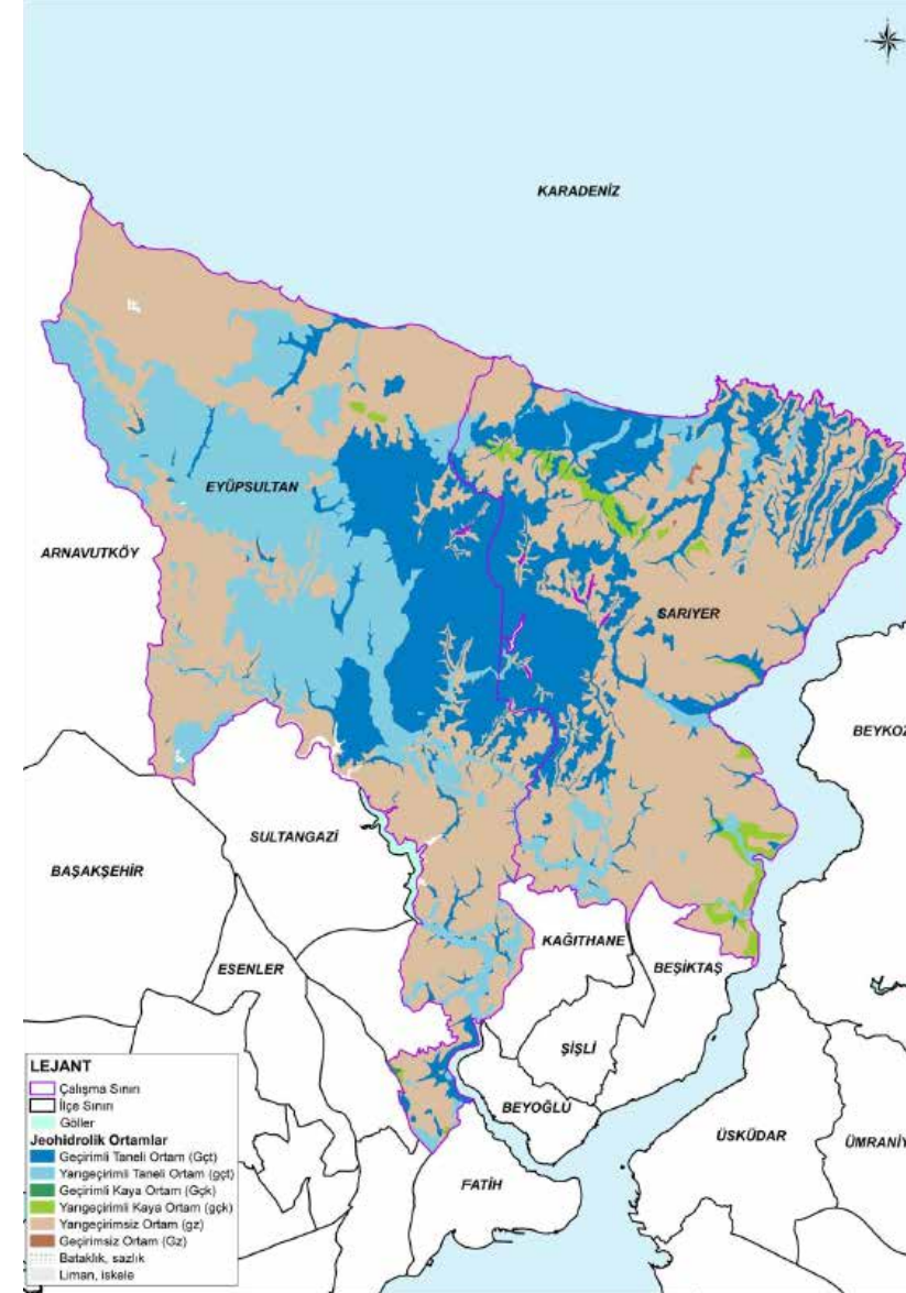
Bölgenin Jeohidrolik Ortamlar Haritası
