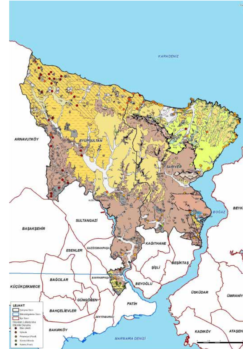
Etkinlik Durumuna Göre Kütle Hareketleri Lokasyonlarının Jeoloji Haritası Üzerinde Gösterimi
