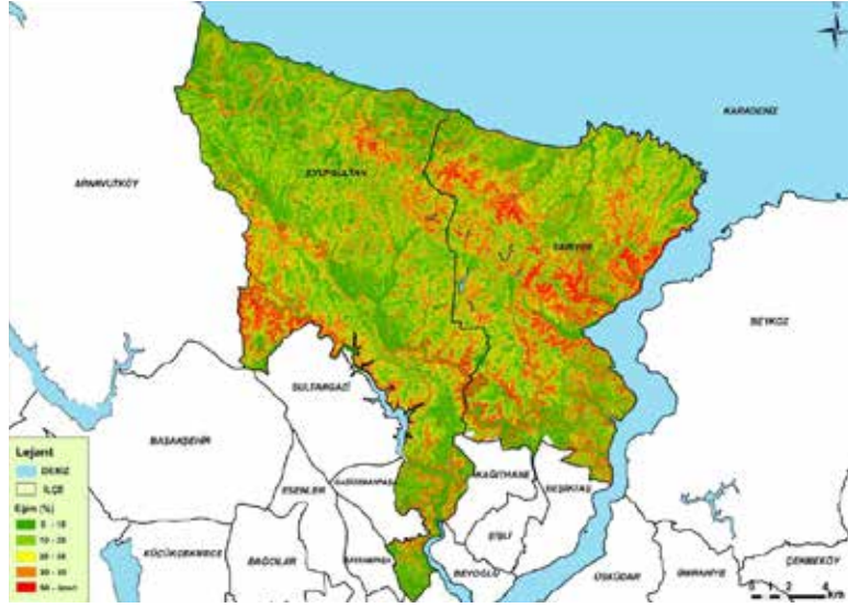
Bölgenin Eğim Haritası
